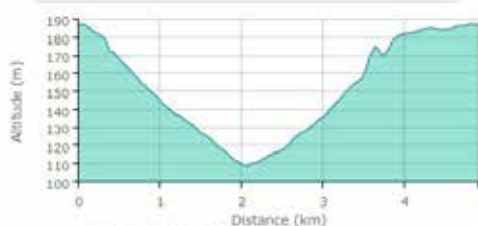
PROFIL ALTIMÉTRIQUE
