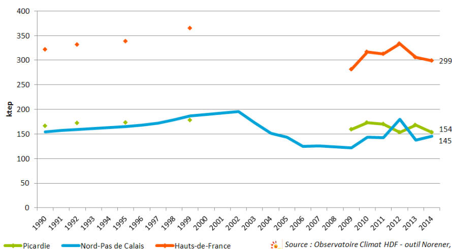
Carte 44. Consommation finale du secteur de l'agriculture Hauts-de-France – Source Observatoire Climat HdF
