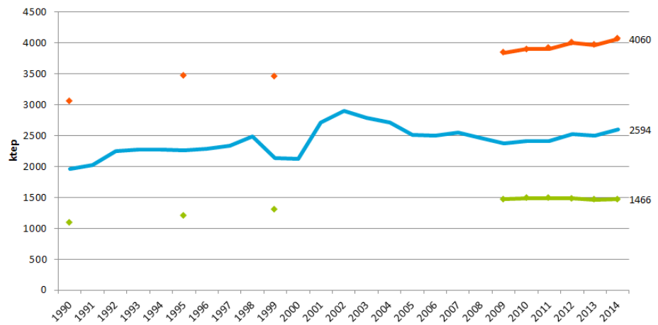
Carte 45. Consommation finale du secteur des transports Hauts-de-France – Source Observatoire Climat HdF
